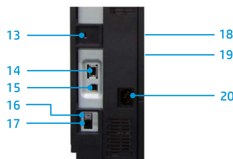
Vue panneau arrière E/S
